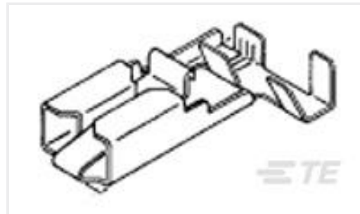
TE Part #926790-4 PL 250 FLAG REC 1-2.5 MM2 PTP CUZN30 F53
