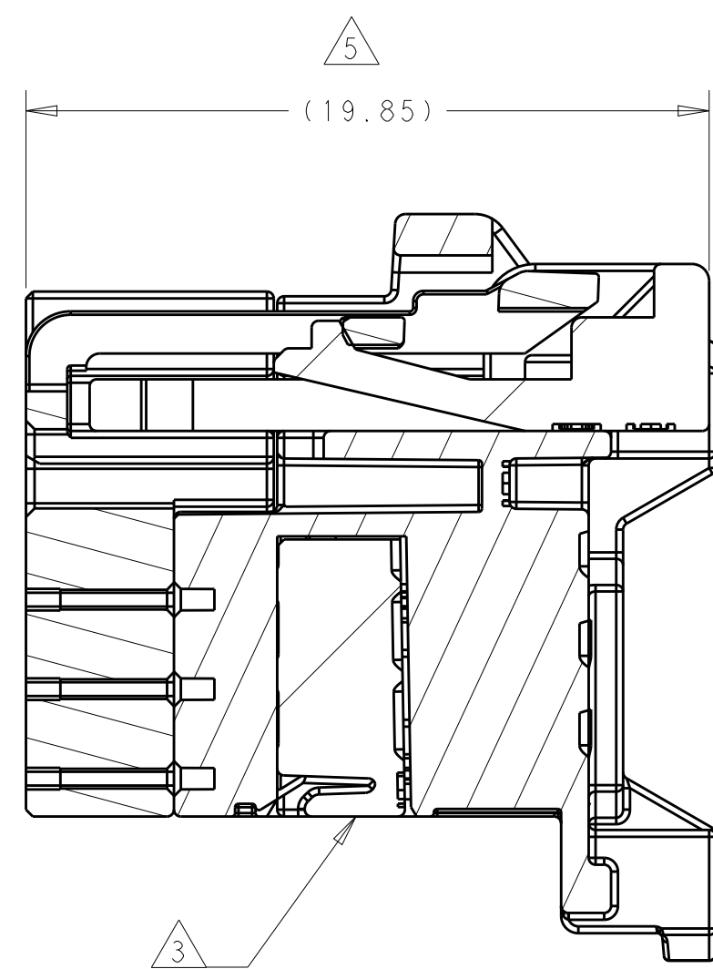
SECTION D-D
