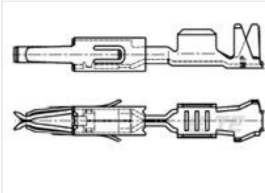
TE Part #964263-3 MT2 A REC 1.6 Contact SRC Au
