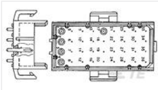
TE Part #2-640500-4 06P MR HDR ASSY VO LF
