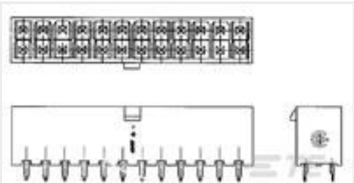
TE Part #1-1586037-0 10P VERT HDR VAL-U-LOK V2
