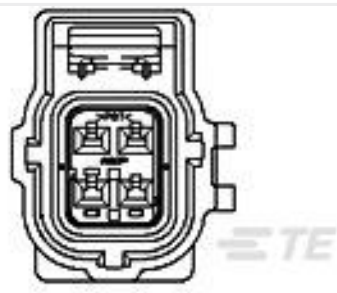
TE Part #184394-1 2X2 PLG ASY W/RET W/O CPA C3-A
