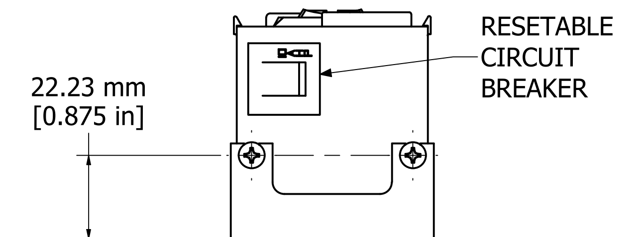
VIEW A-A
