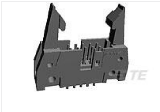
TE Part #5499160-1 A/L UNIV HDR 10P VERT SHT LAT
