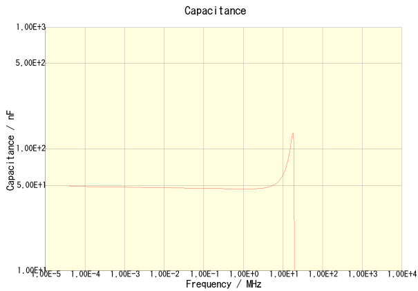
C3216X7R2E473K160AA
