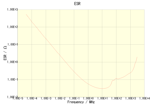
C3216X7R2E473K160AA
