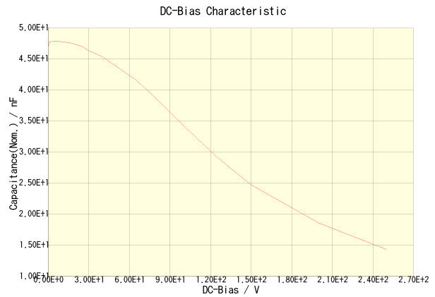
C3216X7R2E473K160AA
