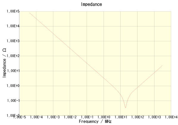
C3216X7R2E473K160AA
