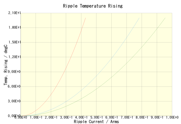
C3216X7R2E473K160AA(100kHz) C3216X7R2E473K160AA(500kHz) C3216X7R2E473K160AA(1MHz)
