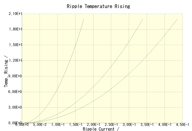
C2012X7R2E103K125AA(100kHz) C2012X7R2E103K125AA(500kHz) C2012X7R2E103K125AA(1MHz)
